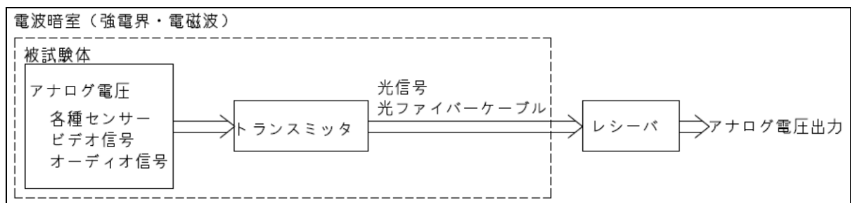
図 1. 暗室からの信号電圧出力:FO-ST,SR
