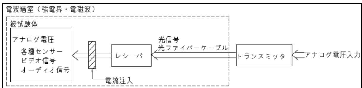
図 2. 暗室への信号電圧入力(BCI テスト):FO-HBST,HBSR
