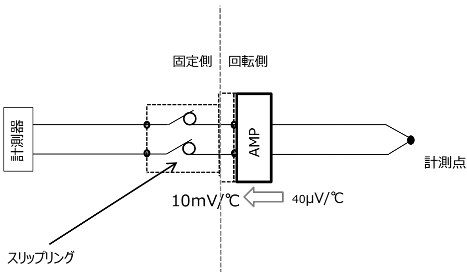
図6. スリップリング+熱電対回転アンプ
